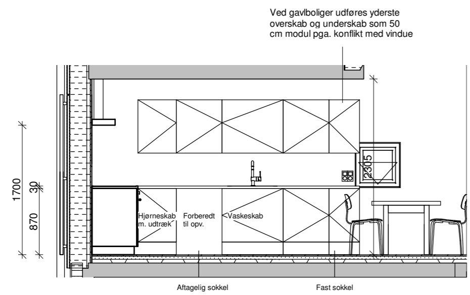
Opstalt A
