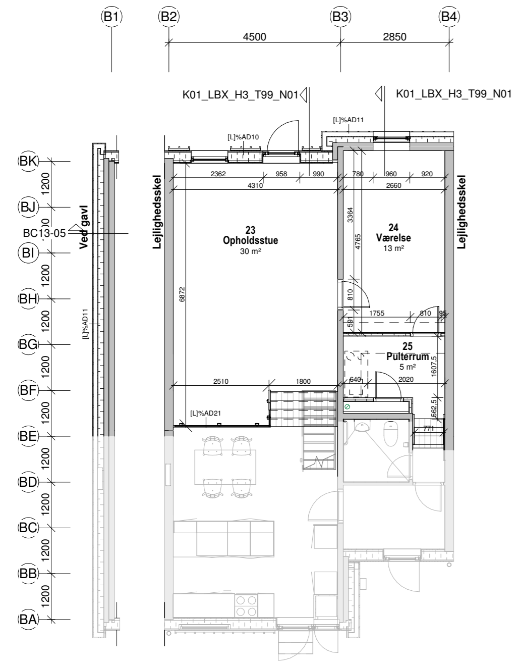
Nedre plan
