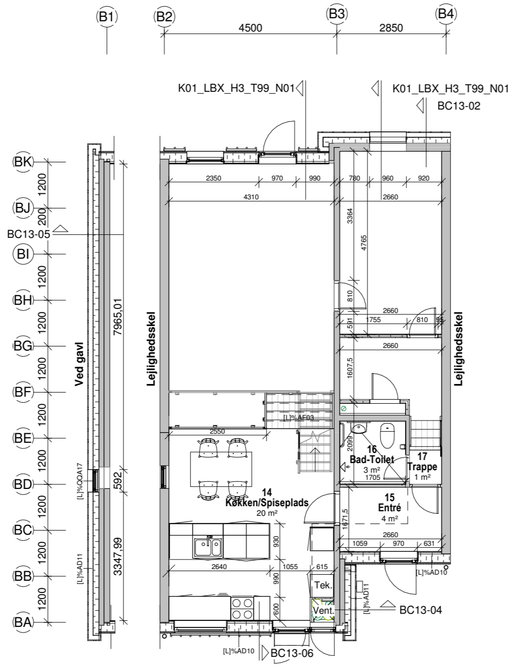
Stueplan
