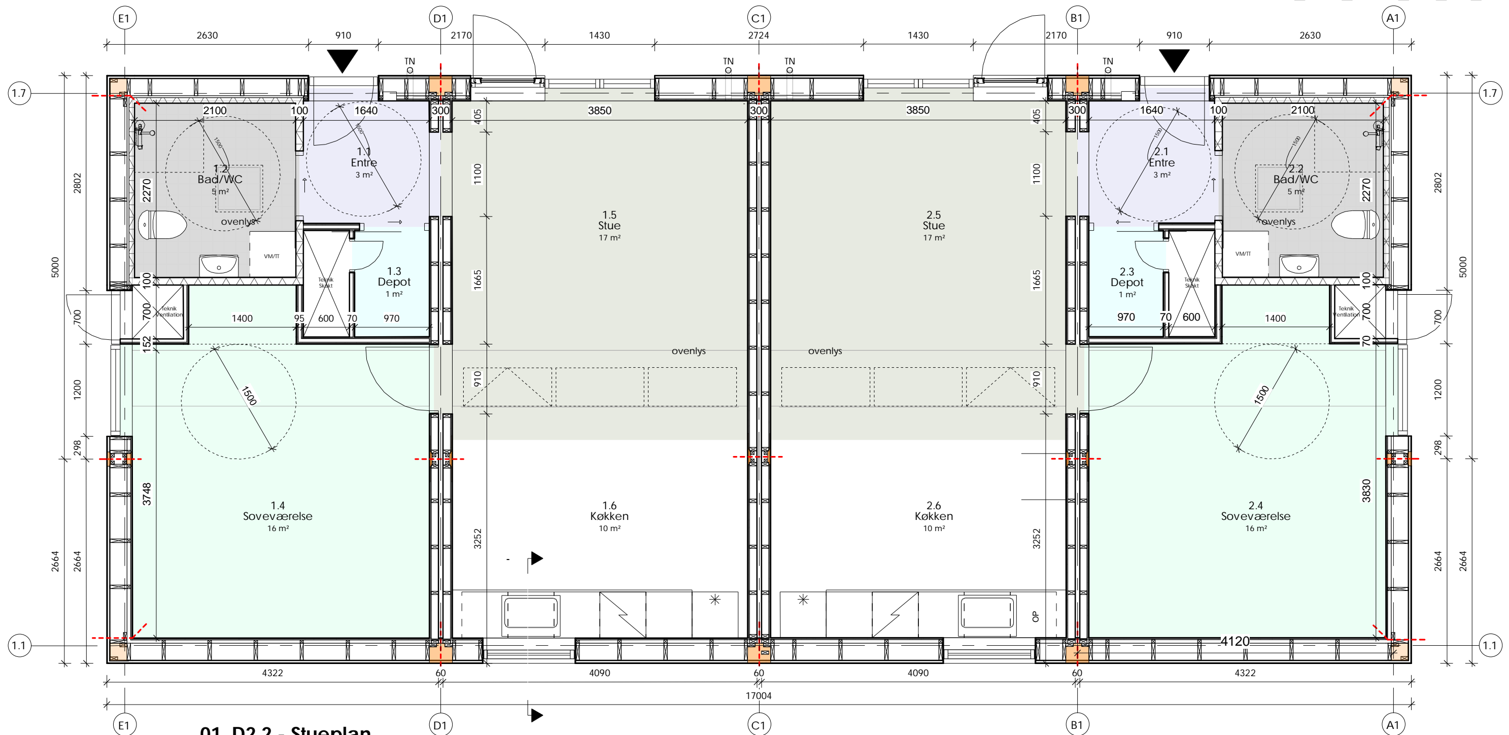
01, D2.2 - Stueplan 1 : 50
