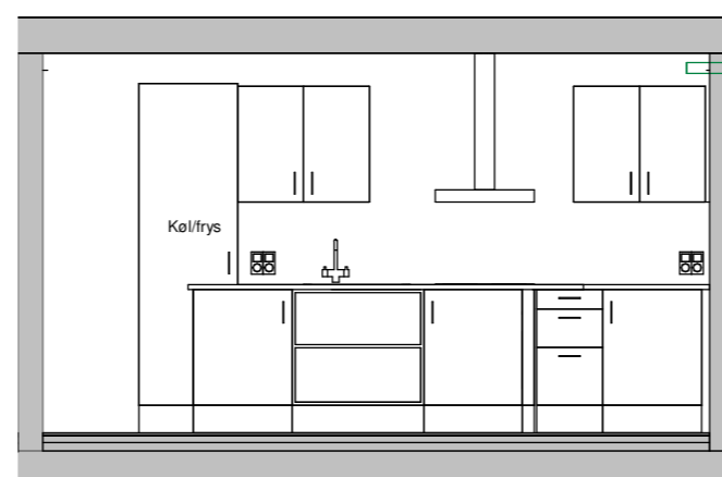
Opstalt A 1 : 50
