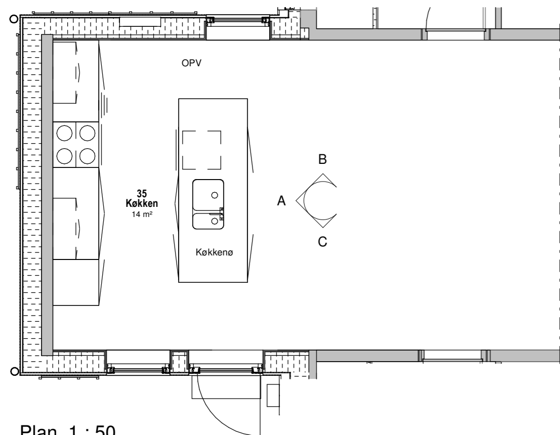
Plan 1 : 50
