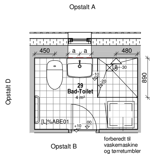
Plan 1 : 50
