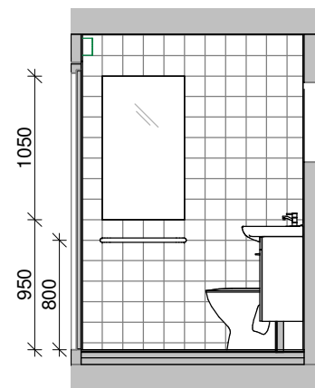
Opstalt D 1 : 50
