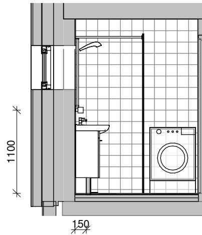
Opstalt C 1 : 50
