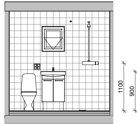
Opstalt A 1 : 50
