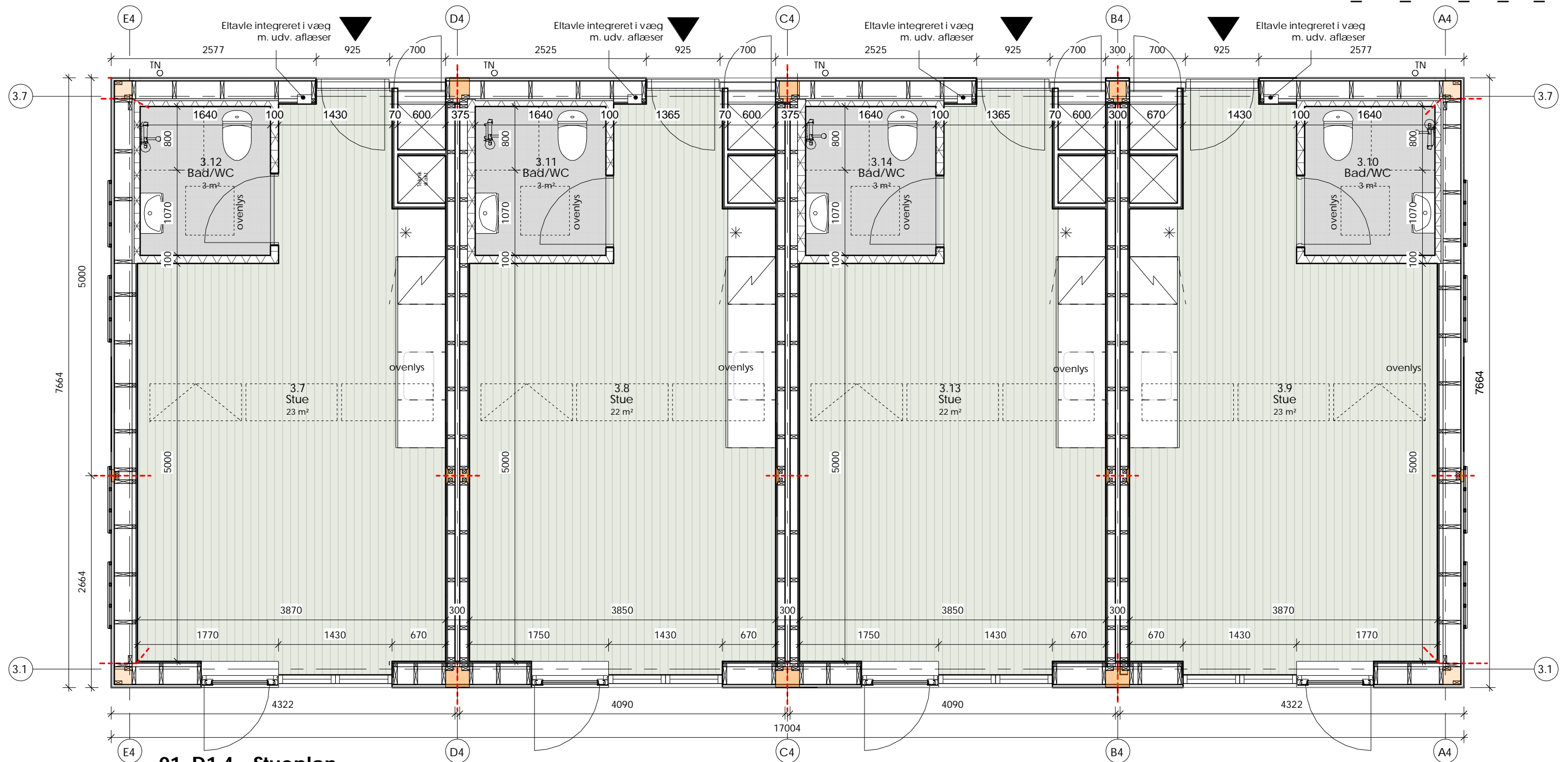
01, D1.4 - Stueplan 1 : 50
